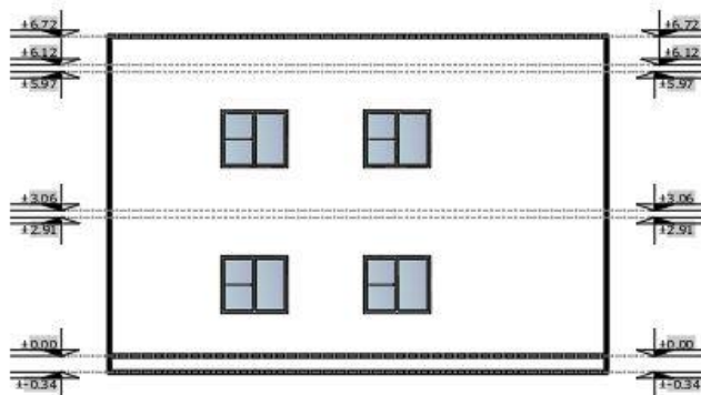
Figura 15. Fasada nga Jugu
